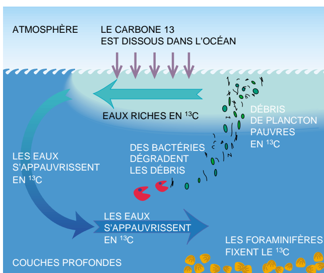
3. LE CARBONE 13 SERT DE MARQUEUR DE LA CIRCULATION OCÉANIQUE. Le dioxyde de carbone de l'atmosphère, se dissout dans les eaux de surface, qui s'enfoncent vers les profondeurs, avec un certain apport de ^{13}\text{C}/^{12}\text{C} . À mesure qu'elles s'éloignent, elles reçoivent des débris de plancton, pauvres en ^{13}\text{C} , dégradés par des bactéries, et s'appauvrissent donc en ^{13}\text{C} .
